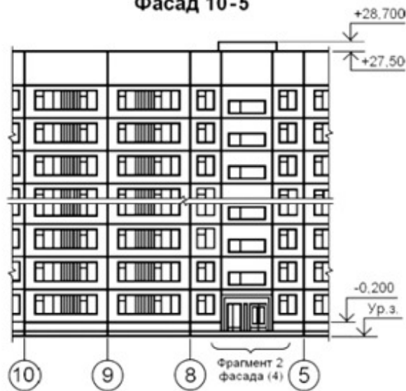
Рисунок Д.2 - Пример выполнения фасада жилого дома
