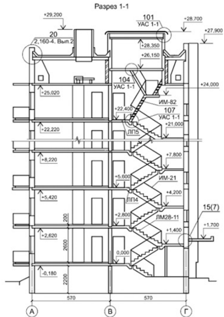
Рисунок Г.3 - Пример выполнения разреза жилого дома
