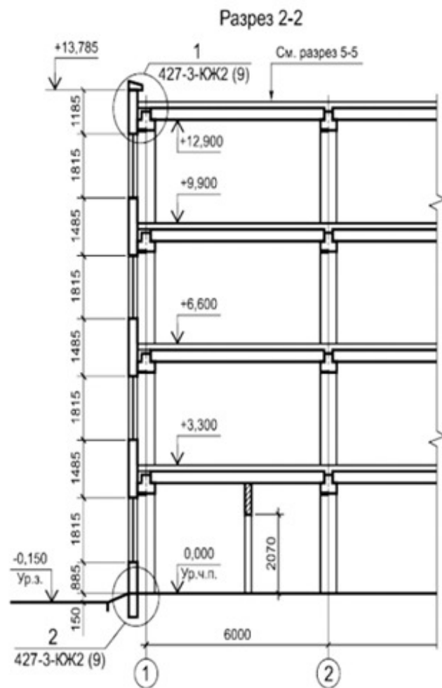
Рисунок Г.2 - Пример выполнения разреза многоэтажного производственного здания
