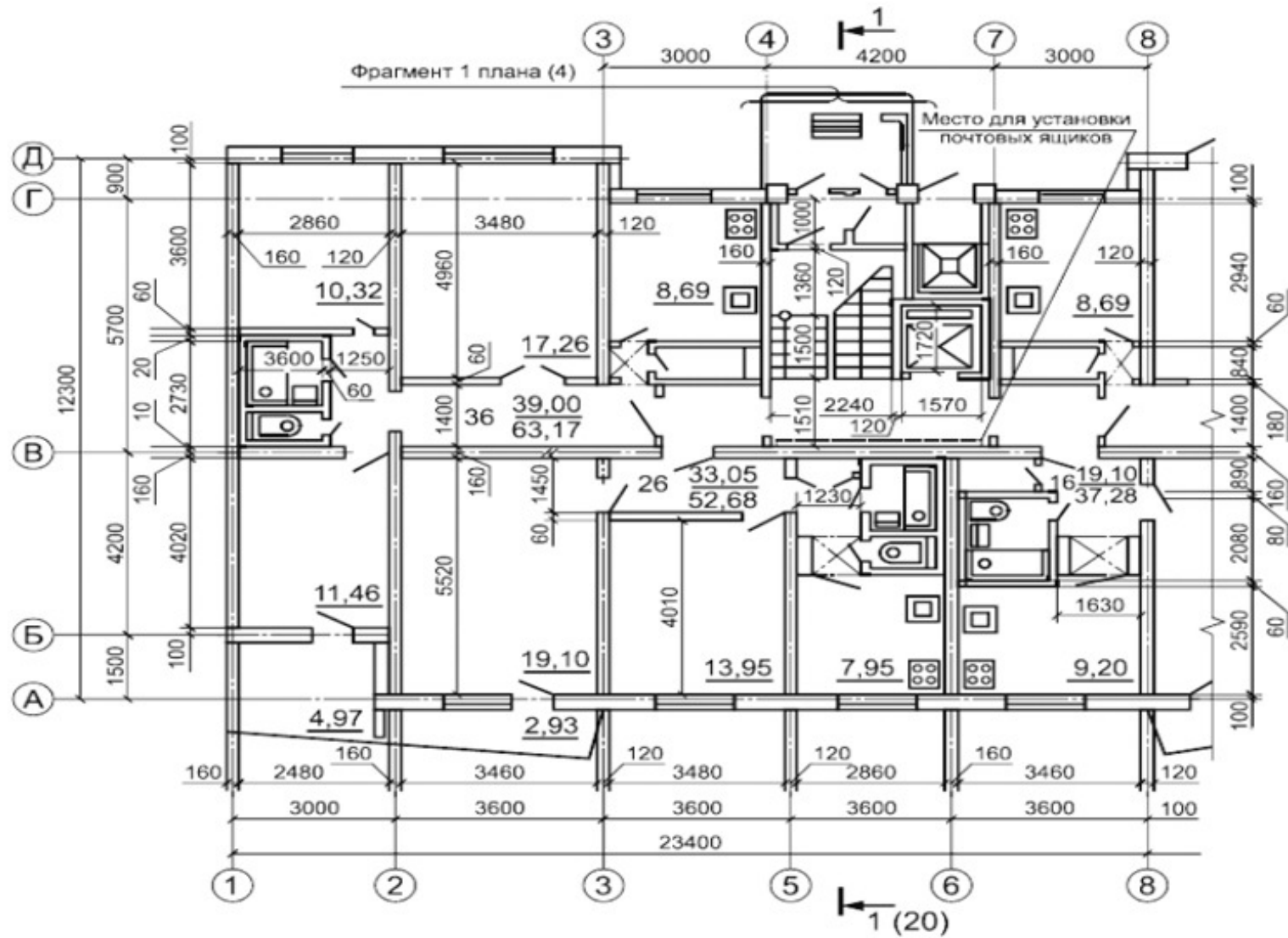
Рисунок Б.1 - Пример выполнения плана одноэтажного производственного здания
