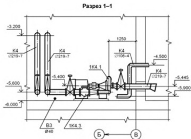
Рисунок В.2 — Пример выполнения разреза установки системы канализации
