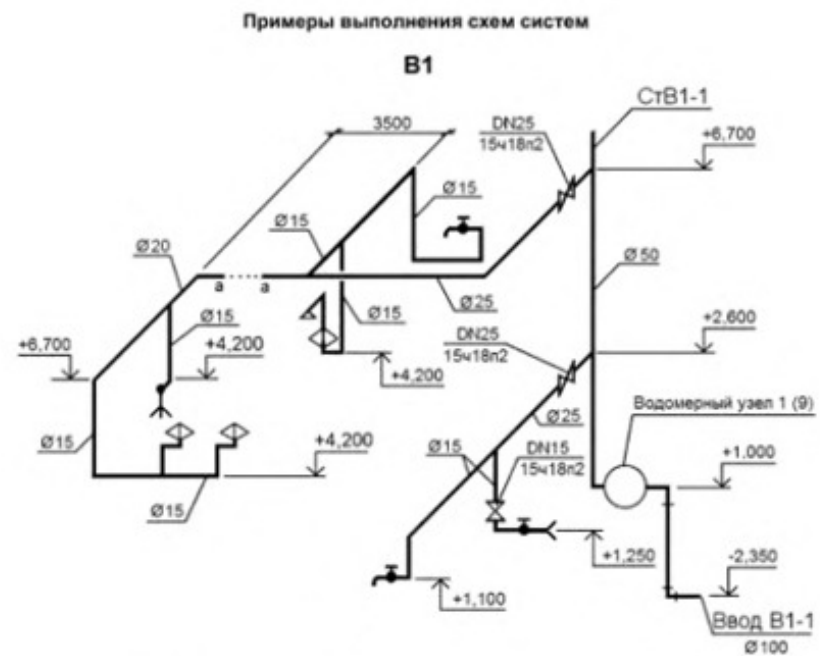
Рисунок Б.1 — Пример выполнения схемы системы водоснабжения
