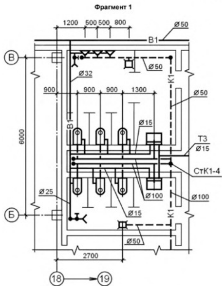
Рисунок А.3 — Пример выполнения фрагмента плана
