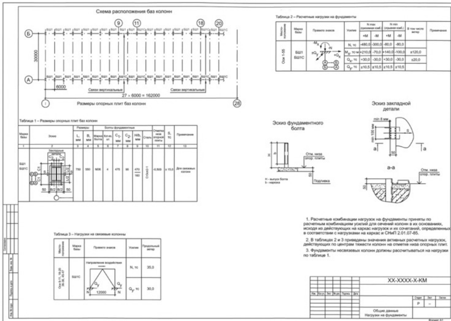
Рисунок В.1 — Пример выполнения нагрузок на фундаменты
